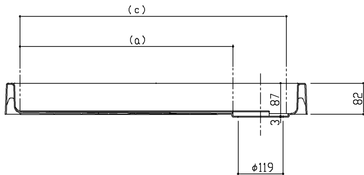
断面A-A
